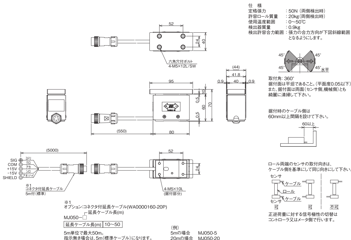
MJ テンションセンサ MODEL MJ050-□ 外形寸法図 図番 MD0000320-JA
