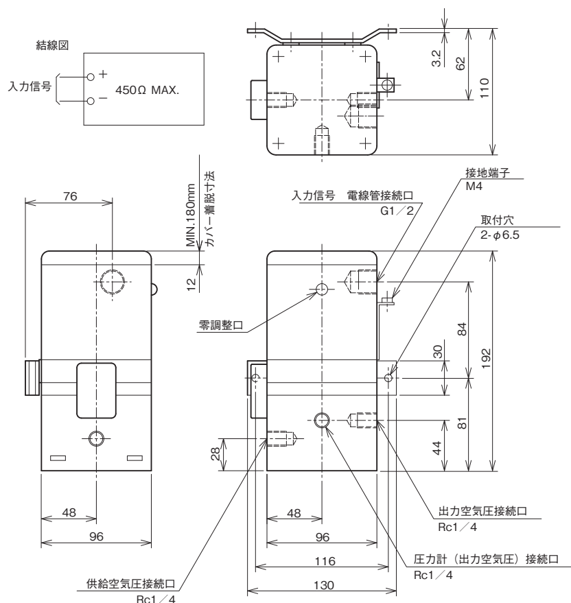
電-空変換器 MODEL EN-40- □□ S-V 本質安全防爆構造 外形寸法図 図番 MD0465.0-JA
