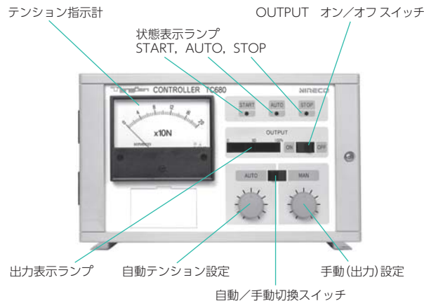
TC680A 前面パネル
