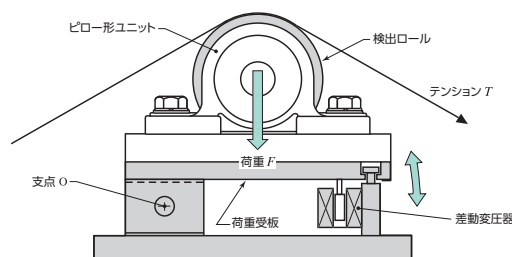
MB25 テンションセンサ構造図
