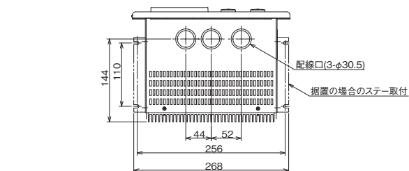
テンションコントローラ MODEL TC680A 外形寸法図 図番 MK0001151-JA
