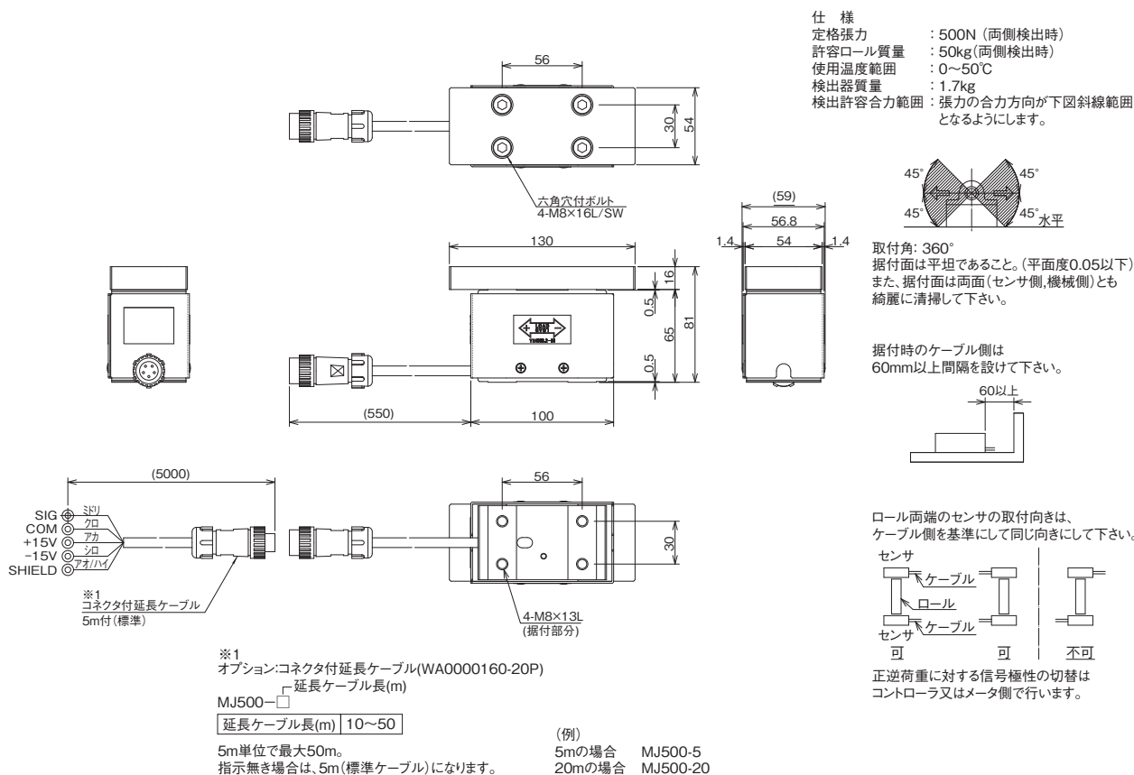
MJ テンションセンサ MODEL MJ500-□ 外形寸法図 図番 MD0000340-JA
