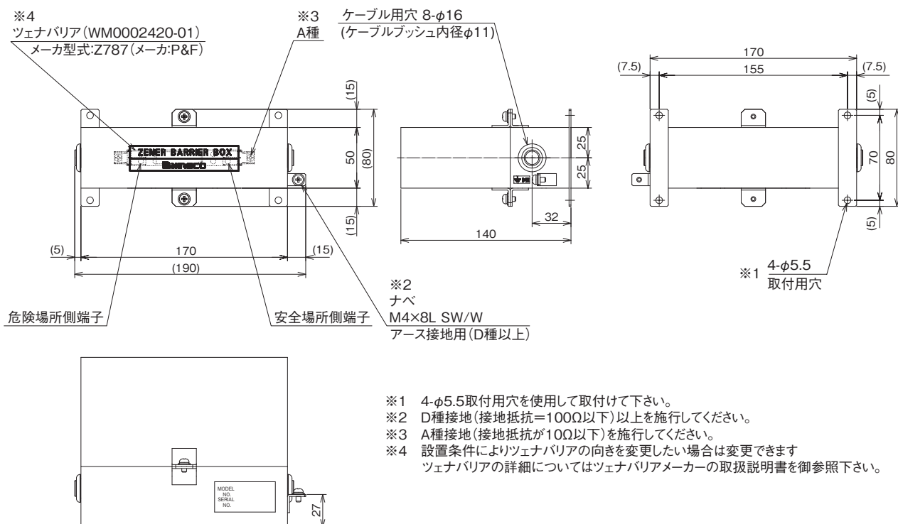
ツェナバリアボックス 本質安全防爆構造 EN40 用 外形寸法図 図番 MK0003590-JA
