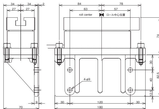
MB25、MB26 □ S 用壁掛けブラケット 外形寸法図 図番 MW1521.0-95P
