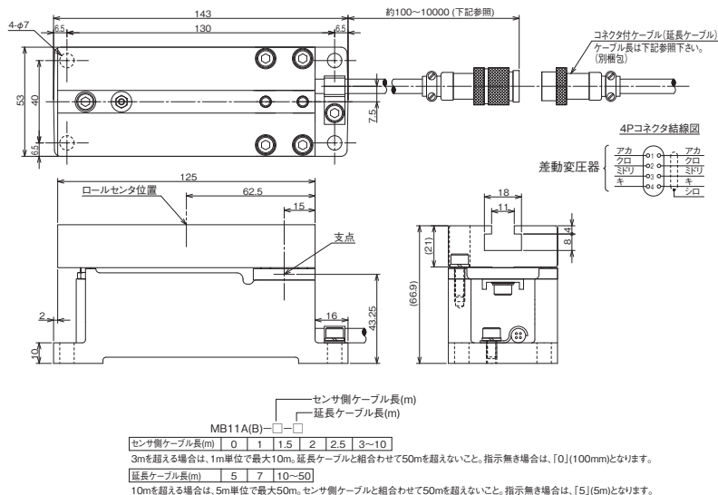
MB テンションセンサ MODEL MB11A-□-□ MB11B-□-□ 外形寸法図 図番 MW1520.0-JA
