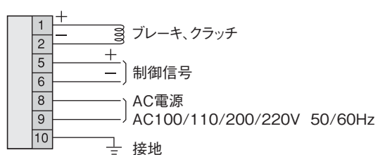
ブースタンプ MODEL TB800 配線図
