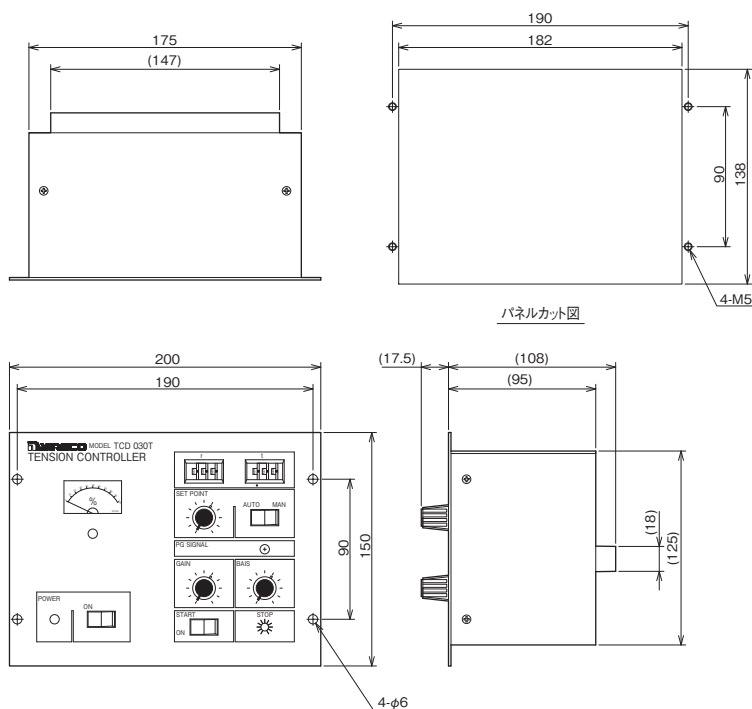
オープンループテンションコントローラ MODEL TCD030T 外形寸法図 図番 MD0004240-JA
