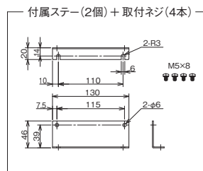
テンションコントローラ MODEL TC680A 外形寸法図 図番 MK0001151-JA
