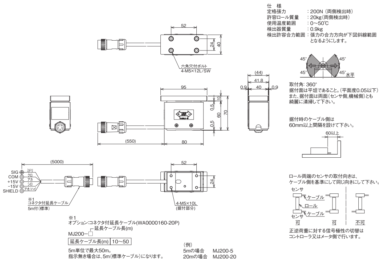
MJ テンションセンサ MODEL MJ200-□ 外形寸法図 図番 MD0000330-JA
