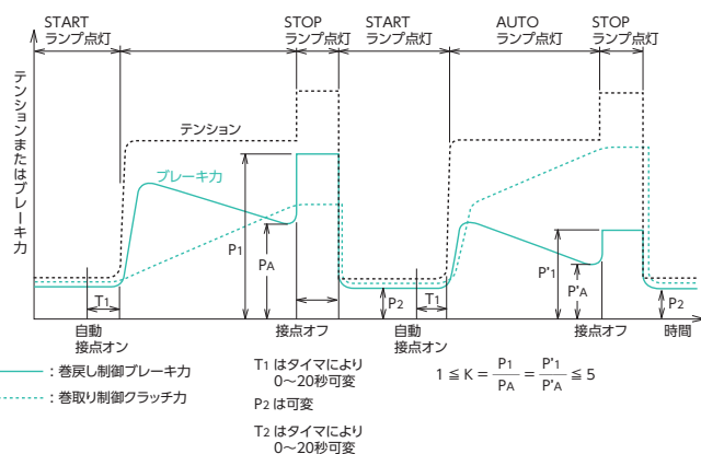
シーケンス動作説明図
