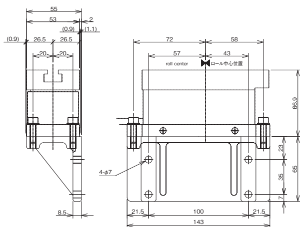
MB11、MB12 □ S 用壁掛けブラケット 外形寸法図 図番 MW1520.0-95P
