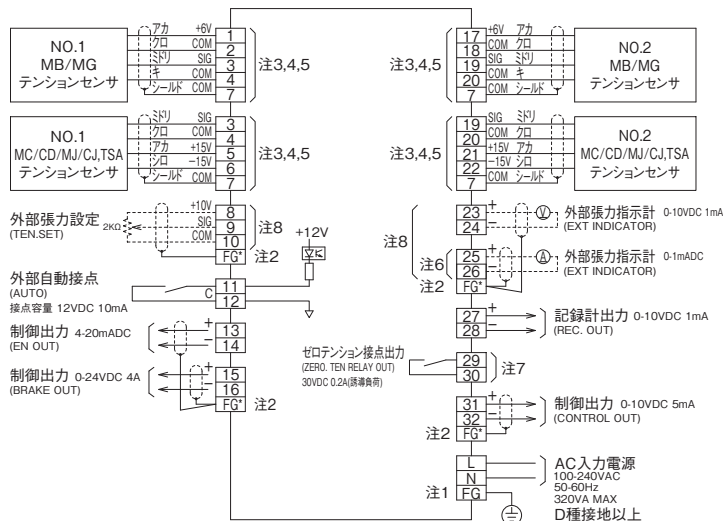
テンションコントローラ MODEL TC680A 配線図 図番 MK0001151-JC
