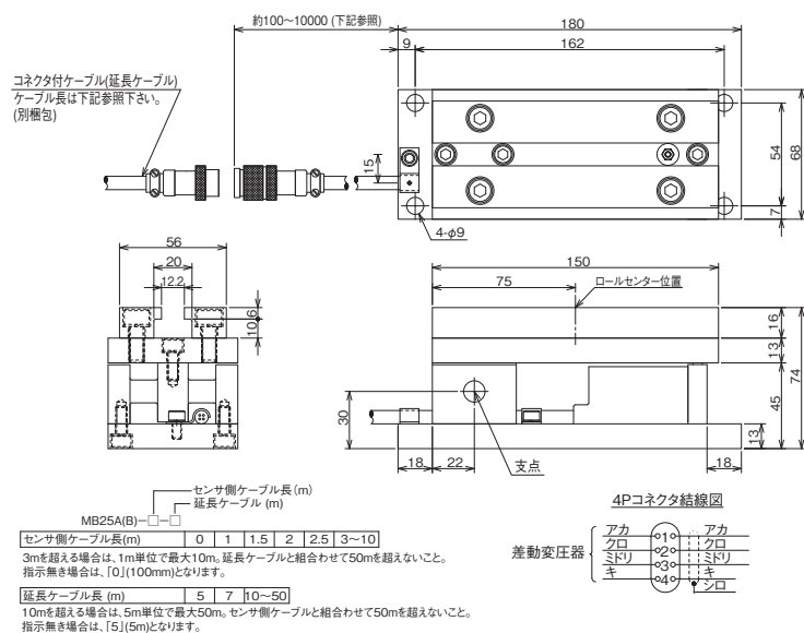
MB テンションセンサ MODEL MB25A-□-□ MB25B-□-□ 外形寸法図 図番 MW1521.0-JA
